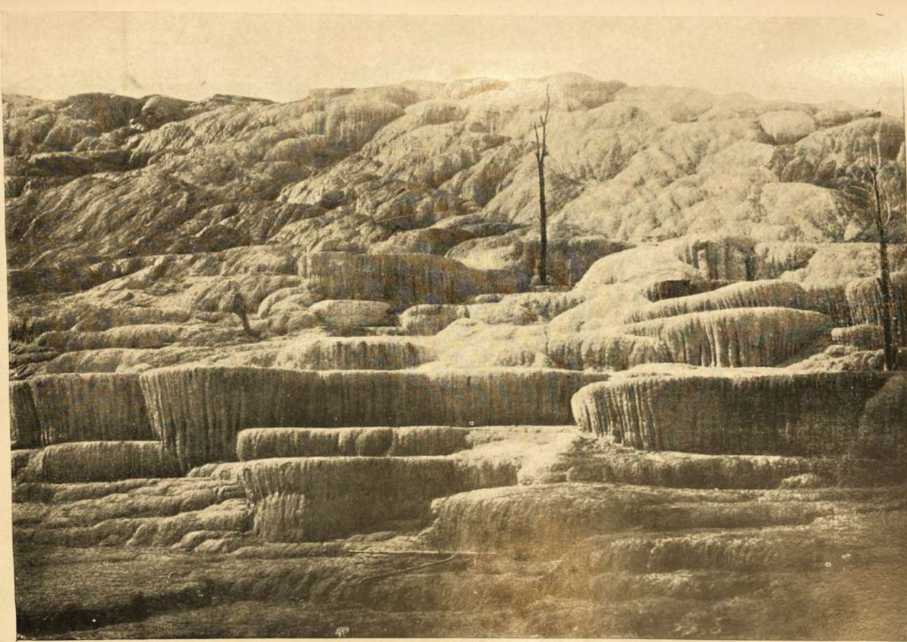
Sorgenti termali incrostanti (carbonato di calcio). Stato di Wyoming, S. U. d'America (Parco Nazionale della Yellowstone).
